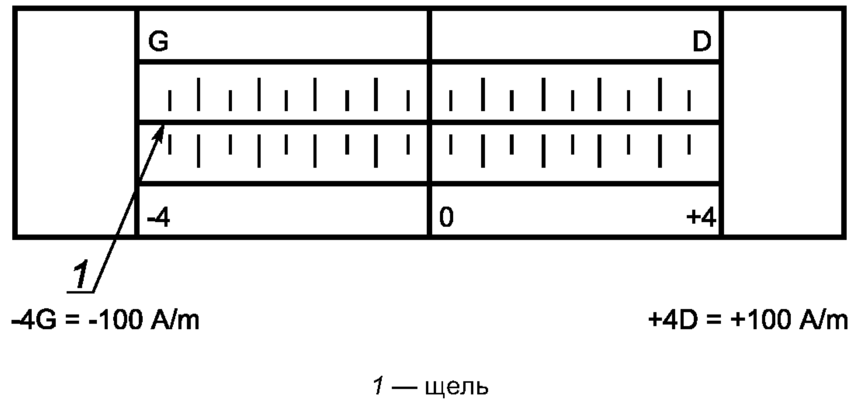
Рисунок В.4 — Гравировка эталонного образца типа 2
