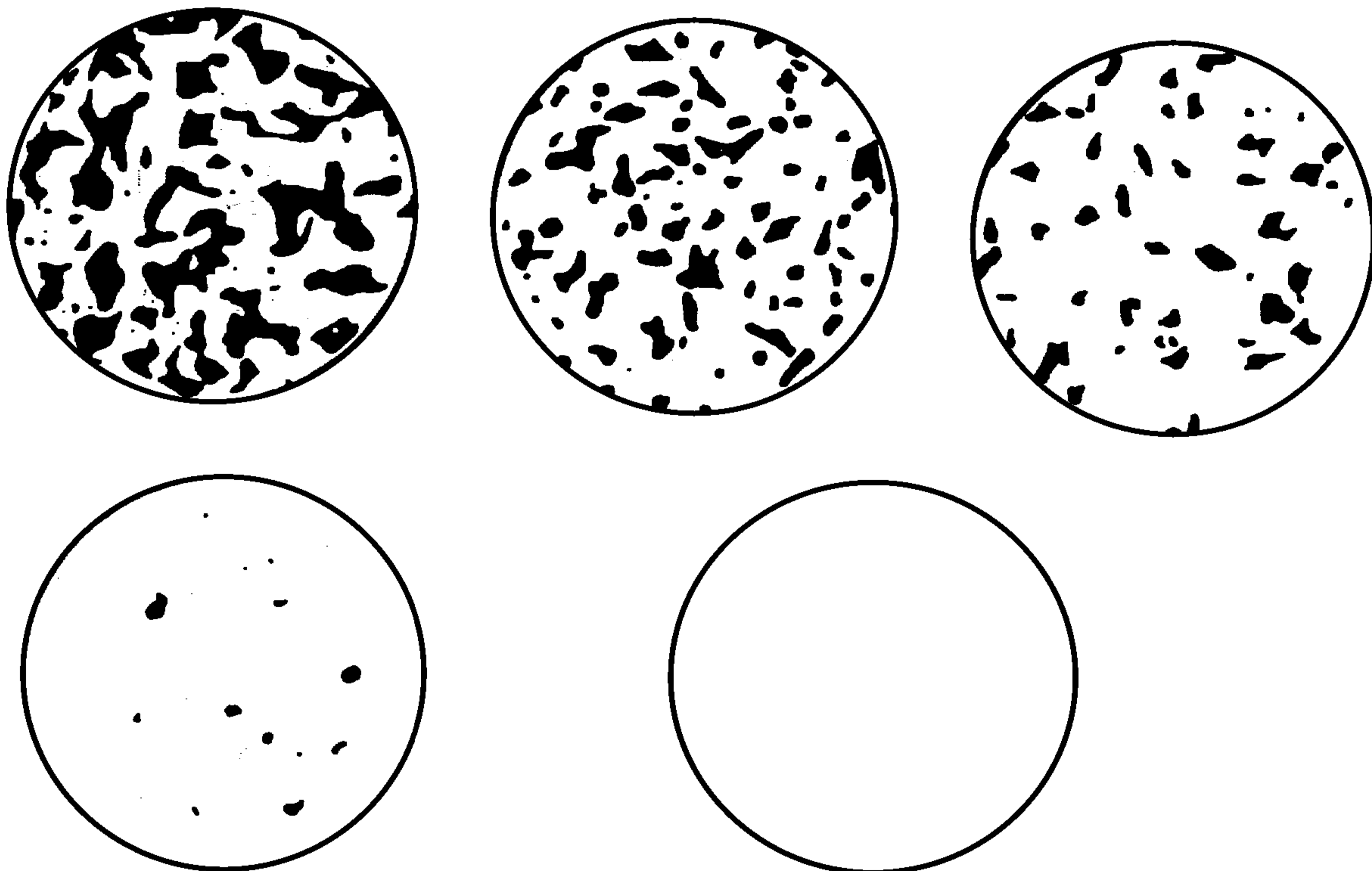
Рисунок С.1 — Оценка следов коррозии
