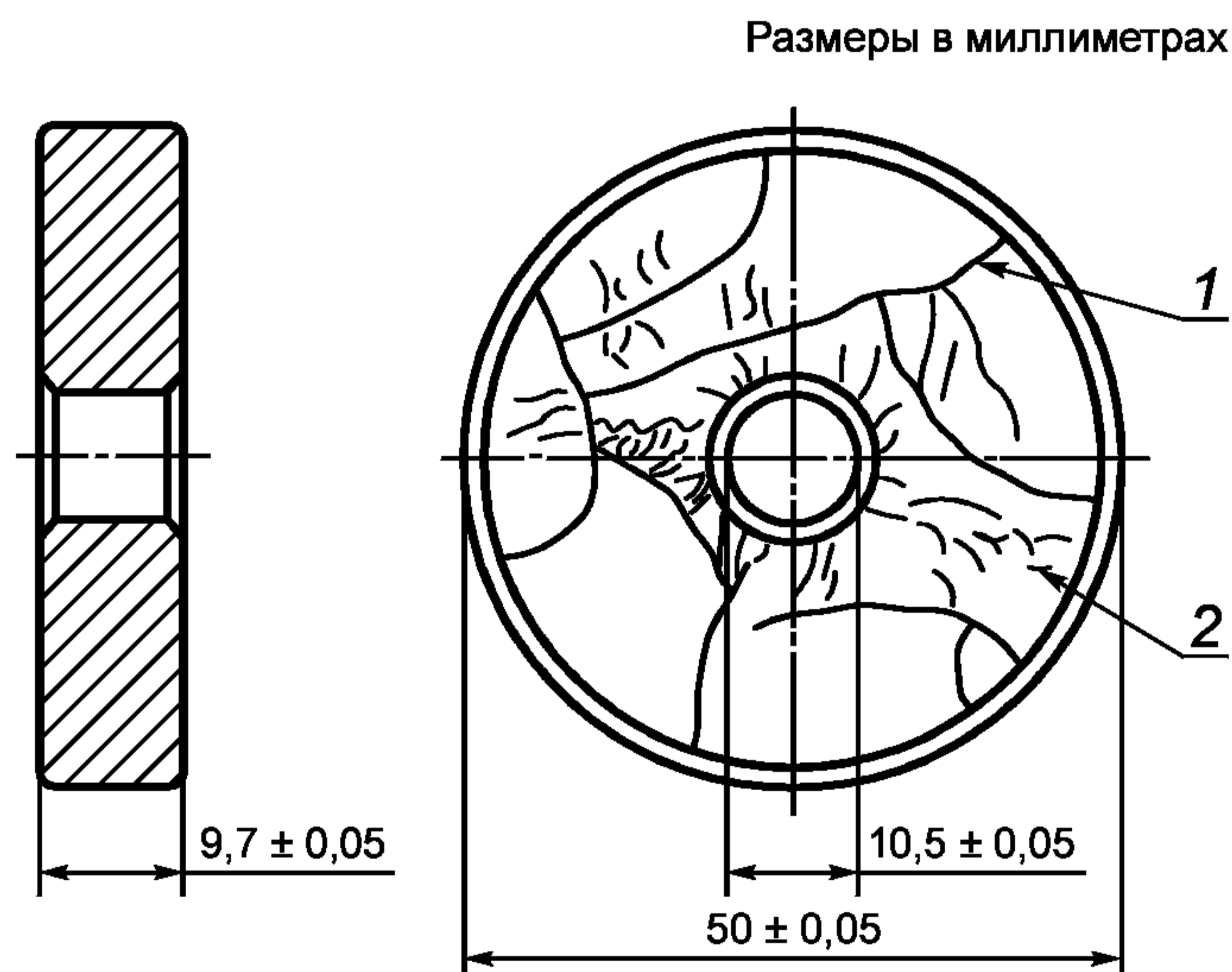
Рисунок В.1 — Эталонный образец типа 1
